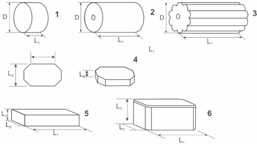
<그림 1> 연료용 목재브리켓의 형태 표시 방법
